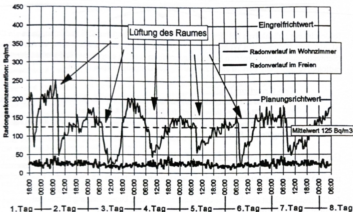
Abb.: Beispiel für die in einem Einfamilienhaus im Mühlviertel gemessene Radongaskonzentration (aktive Meßmethode)
