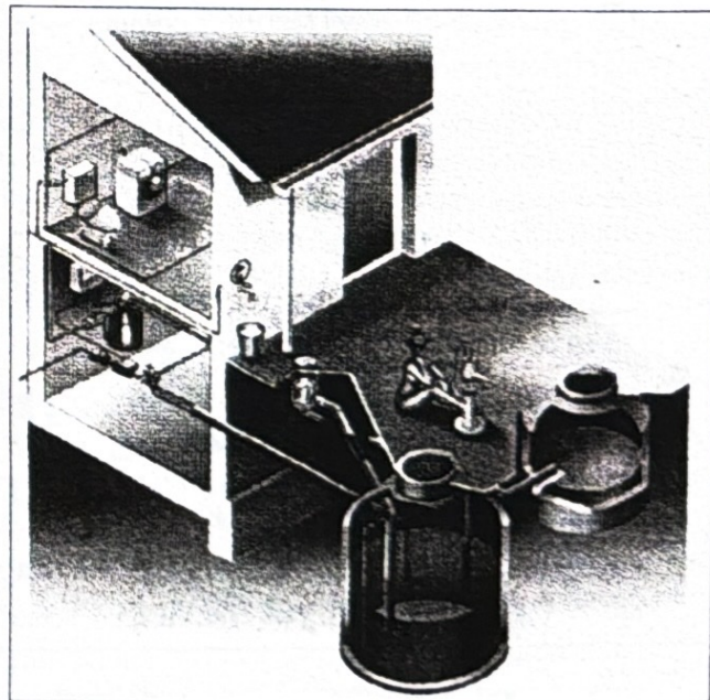
Unter der Handpumpe verbirgt sich die Regenwasser-Nutzungsanlage. Damit lassen sich bis zu 50 Prozent des Trinkwassers einsparen - zur Freude der Familie, der Umwelt und der Brieftasche
